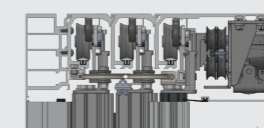
Cajón telescópico 3H 120 x 357 mm
